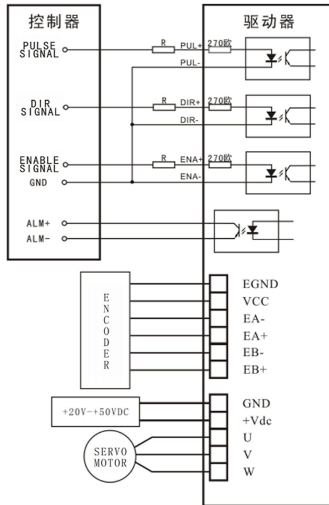
Рисунок 3. Типовая схема подключения драйвера для трёхфазного серво-шагового двигателя.
