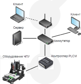
Рис. 8 Вариант развертывания системы в локальной сети
