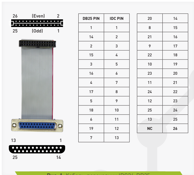
Рис. 1. Кабель-переходник IDC26-DB25
