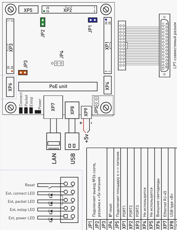
Рис. 2. Схема подключения
