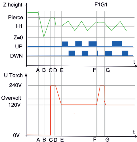
Рис. 3 Графики высоты резака и напряжения дуги
