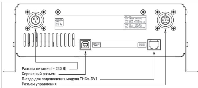
Рис. 5 Вид сзади модуля управления THC2-M
