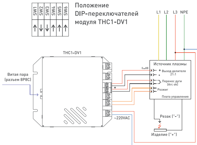
Рис. 7 Подключение к АПР, оборудованному делителем напряжения 25:1 или 50:1 (диапазон измерения 0..8В и 0..4В). АПР подключен ко входу LV блока делителя (см. наклейку на блоке).
