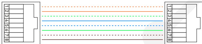
Рис. 6 Схема межблочного кабеля
