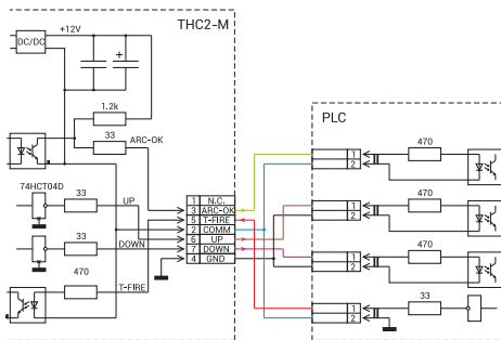
Рис. 10 Подключение THC2-M к плате коммутации.
