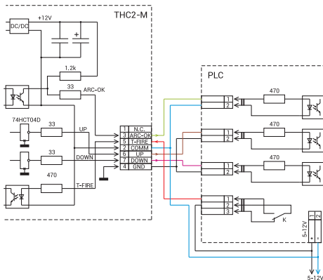
Рис. 11 Подключение THC2-M к плате коммутации с использованием реле.
