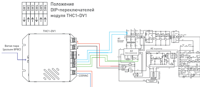
Рис. 9 Подключение к АПР ПУРМ-180, не оборудованному делителем напряжения и без выхода Arc ок (с трансформатором тока).
