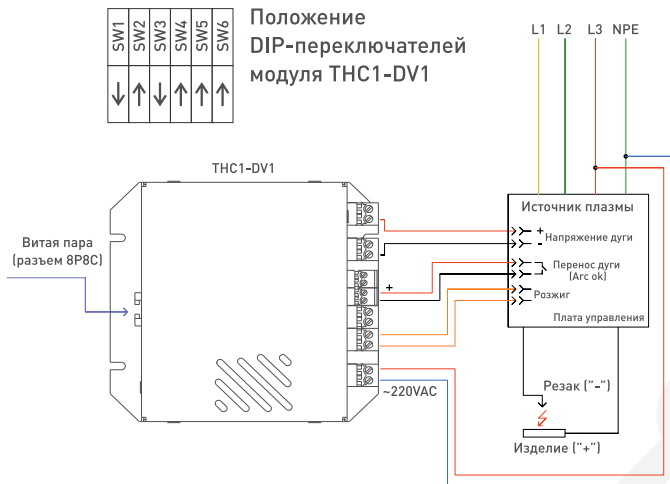
Рис. 8 Подключение к источнику плазмы без делителя напряжения.
