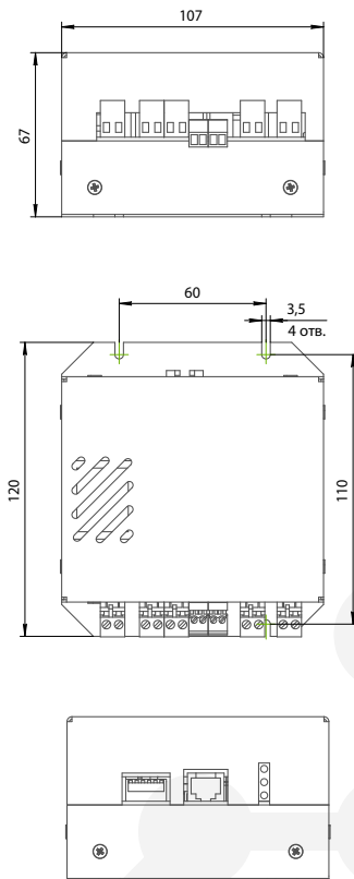
Рис. 2 Габаритный чертеж модуля делителя напряжения THC1-DV1
