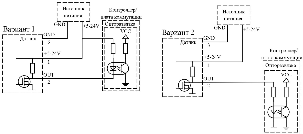
Рисунок 3 - Варианты подключения устройства.
