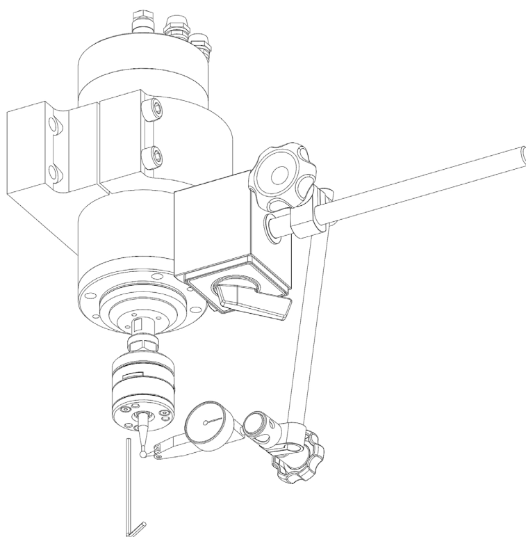
Рисунок 4 - Юстировка датчика.
