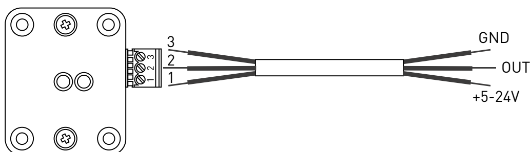
Рисунок 2 - Подключение модуля датчика.
