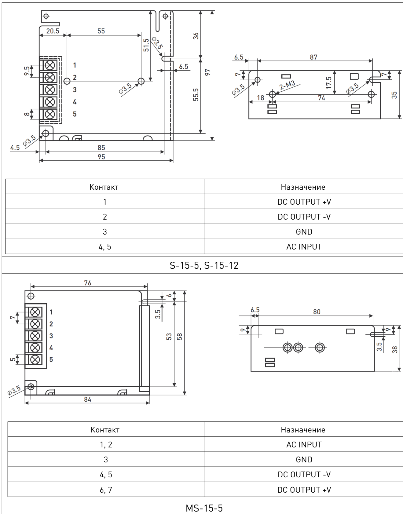
Рис. 2. Габаритные и установочные размеры источников питания
