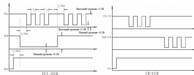
Рис. 11. Схема последовательности управляющих сигналов
