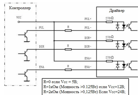
Рис. 3. Подключение к выходам "открытый коллектор" (с общим анодом)
