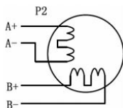
Рис. 5. Схема подключения двигателя с 4 выводами
