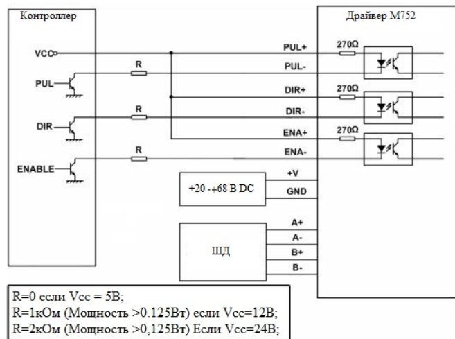
Рис. 10. Типовая схема подключения
