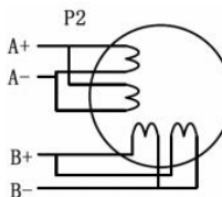
Рис. 9. Схема параллельного подключения двигателя с 8 выводами
