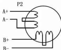
Рис. 8. Схема последовательного подключения двигателя с 8 выводами
