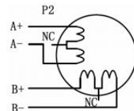
Рис. 7. Подключение двигателя с 6 выводами (полная обмотка, высокий момент)
