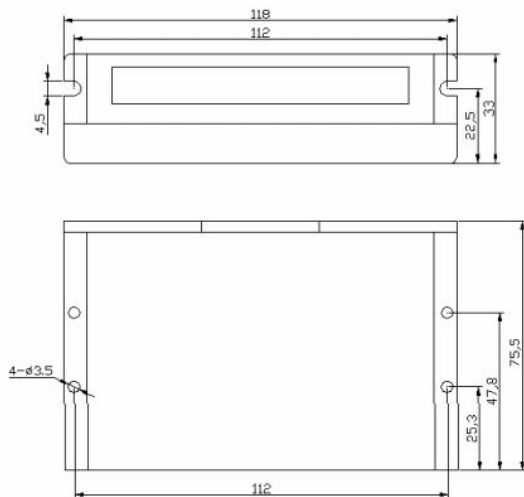
Рис. 1. Механически характеристики
