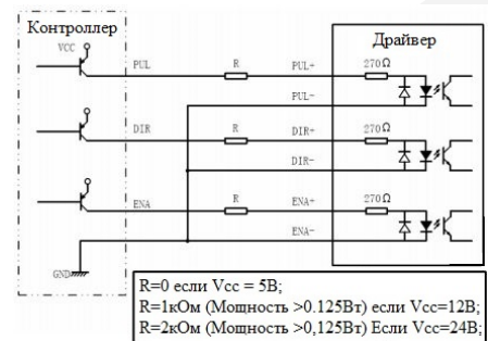
Рис. 4. Подключение к выходам PNP (с общим катодом)
