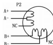
Рис. 6. Подключение двигателя с 6 выводами (полуобмотка, высокая скорость)
