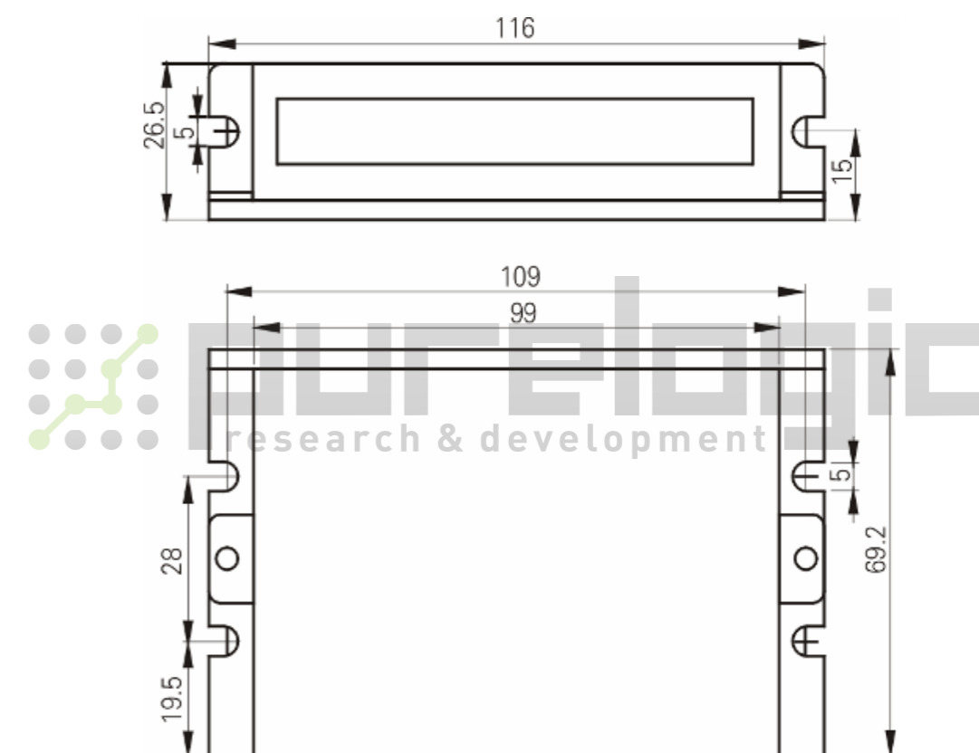
Рисунок 3: Размеры устройства
