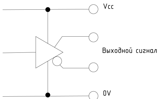
Рисунок 1 - Схема подключения выходов пульта
