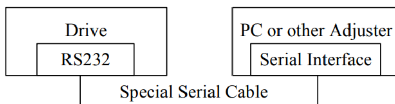
Рисунок 7 – Схема подключения драйвера к внешним устройствам по интерфейсу RS232.
