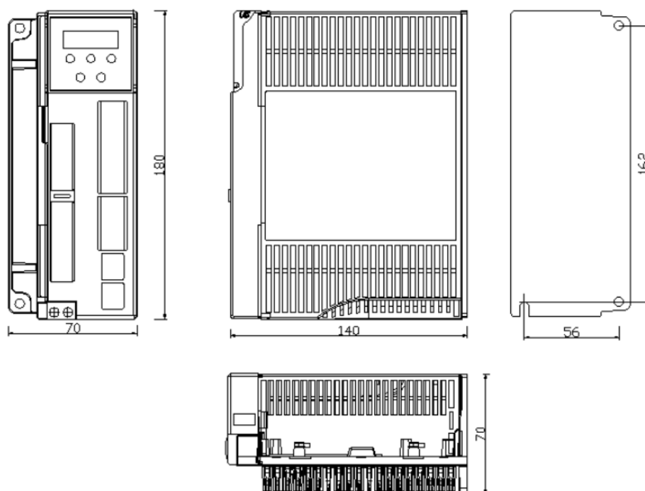
Рисунок 1— Габаритные размеры драйвера 3HSS2208H-130-2500.
