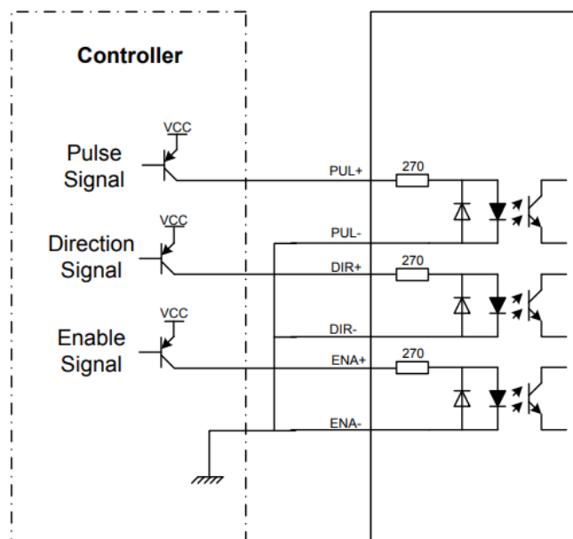
Рисунок 3 — Типовая схема подключения драйвера 3HSS2208H-130-2500 с общим анодом.
