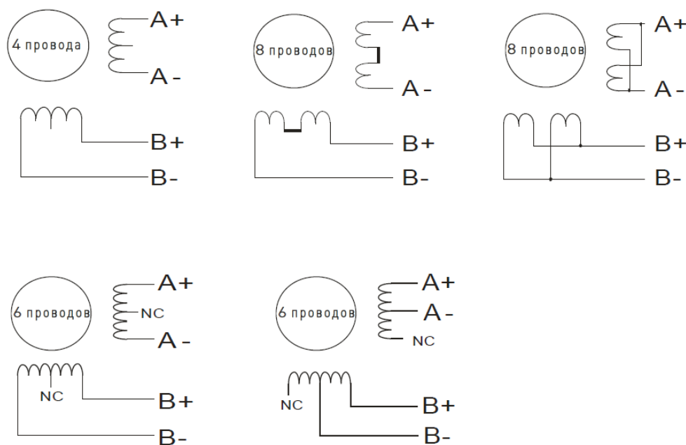
Рисунок 2 — Схема подключения двигателей с 4, 6 и 8 проводами.
