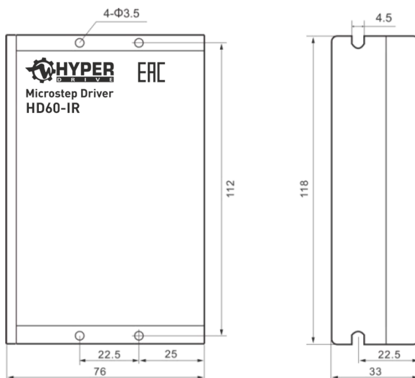
Рисунок 1 — Габаритные характеристики драйвера.
