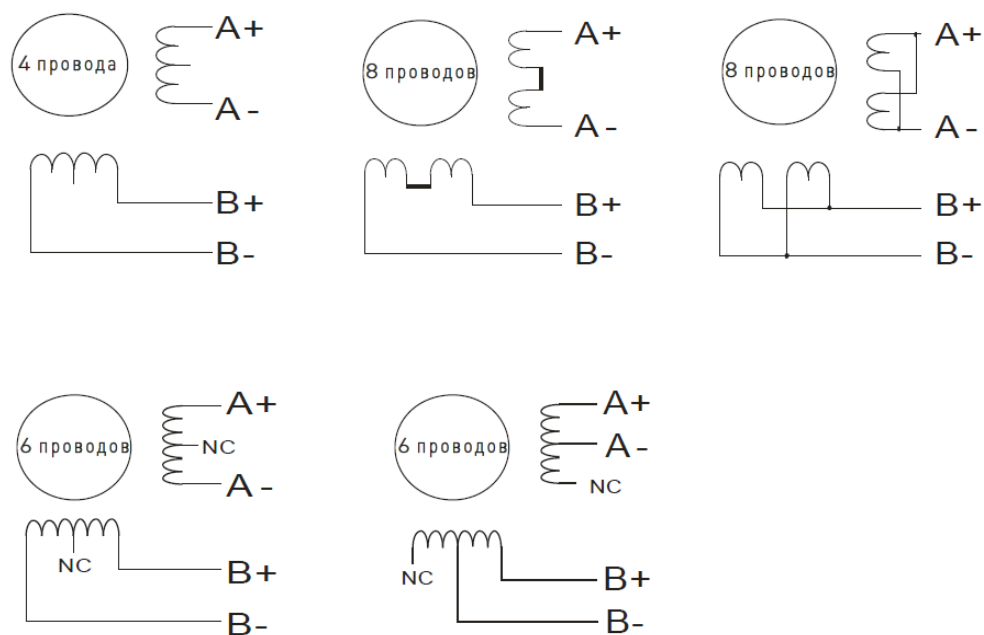
Рисунок 3 — Схема подключения двигателей с 4, 6 и 8 проводами.
