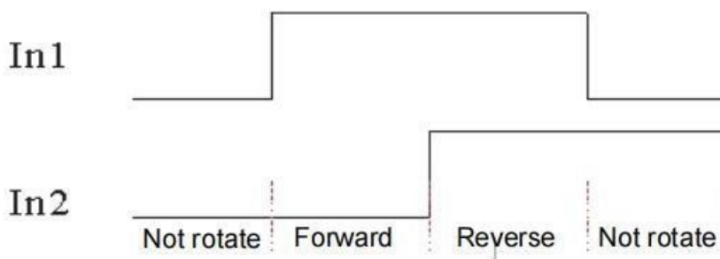
Рисунок 4 — Схема последовательности сигналов при старте/остановке двигателя.
