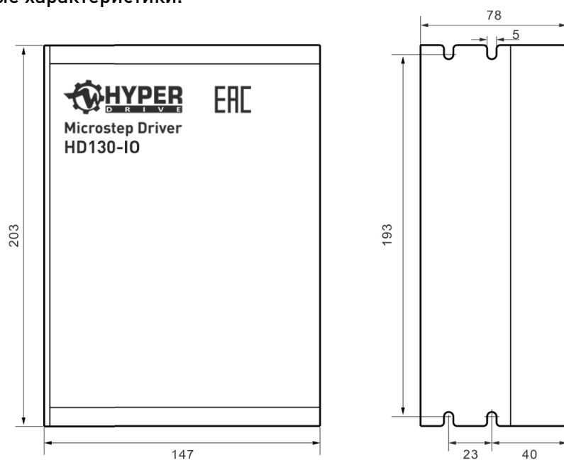
Рисунок 1 — Габаритные характеристики драйвера.
