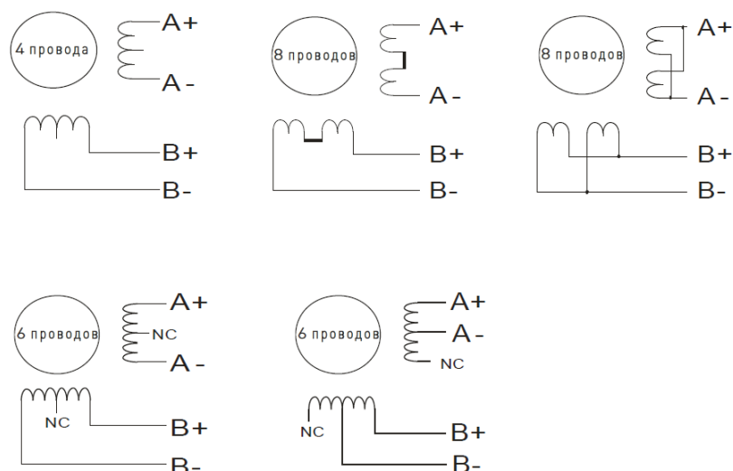
Рисунок 2 — Схема подключения двигателей с 4, 6 и 8 проводами.
