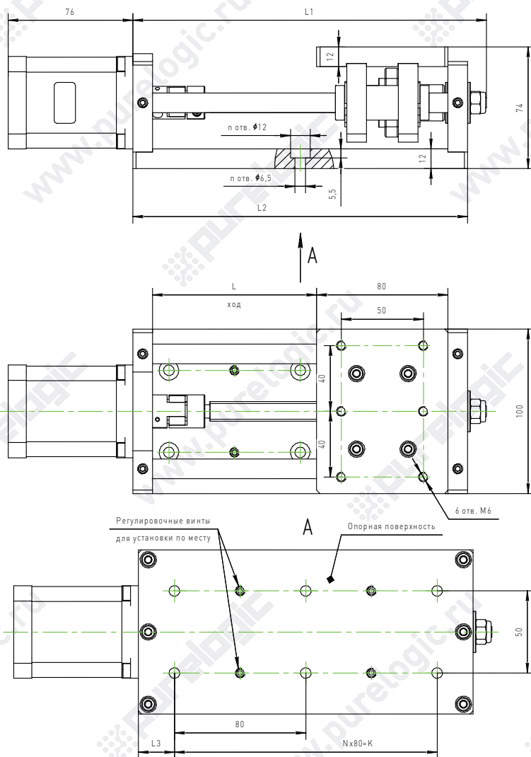
Модуль линейного перемещения PLLM-01
