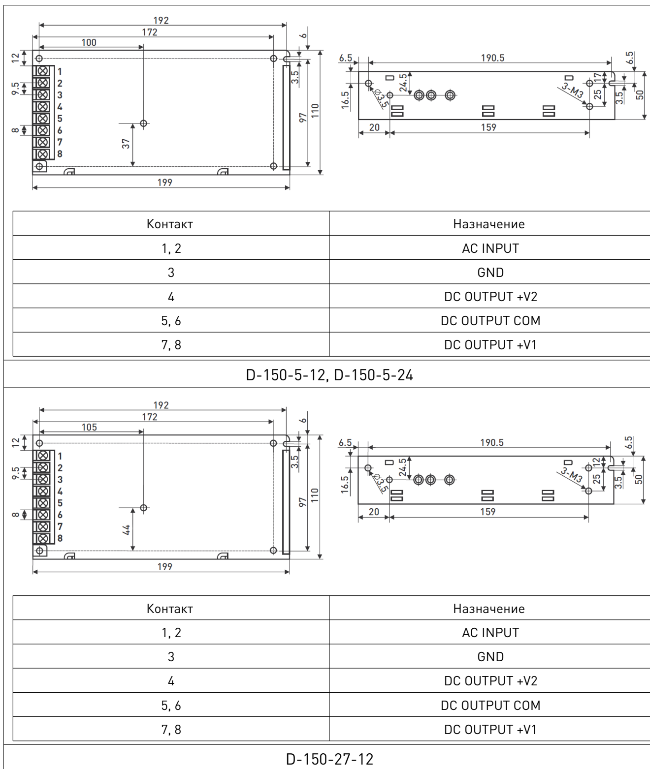
Рис. 2. Габаритные и установочные размеры источников питания
