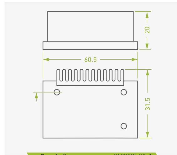
Рис. 1. Размеры модуля SU3235-02-1
