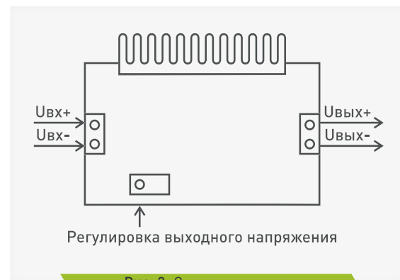
Рис. 2. Схема подключения
