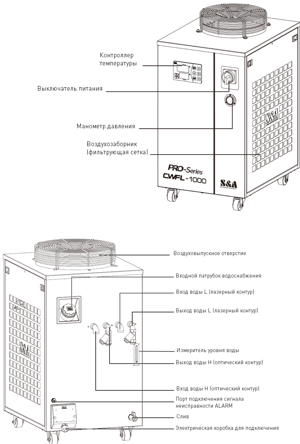
Рисунок 1 – Внешние элементы чиллера.
