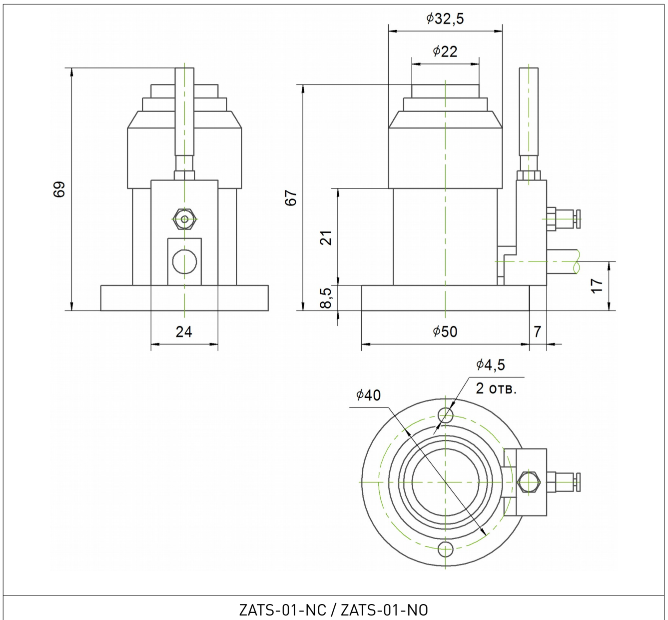
Рис. 2. Габаритные и установочные размеры датчика высоты инструмента
