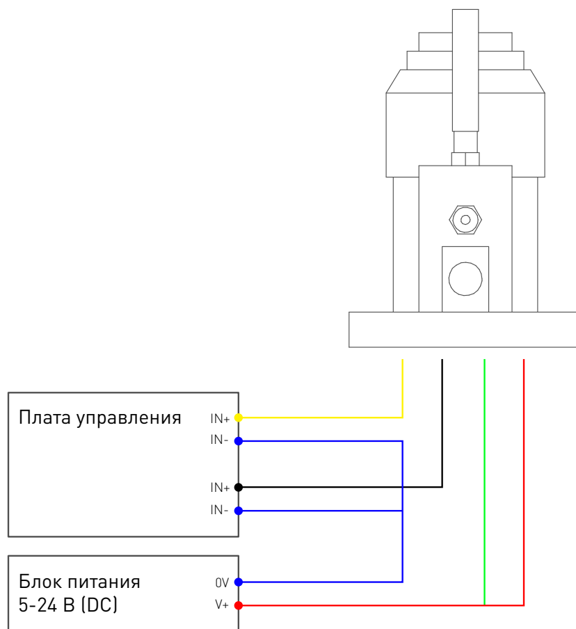
Рис. 3. Подключение датчика высоты инструмента
